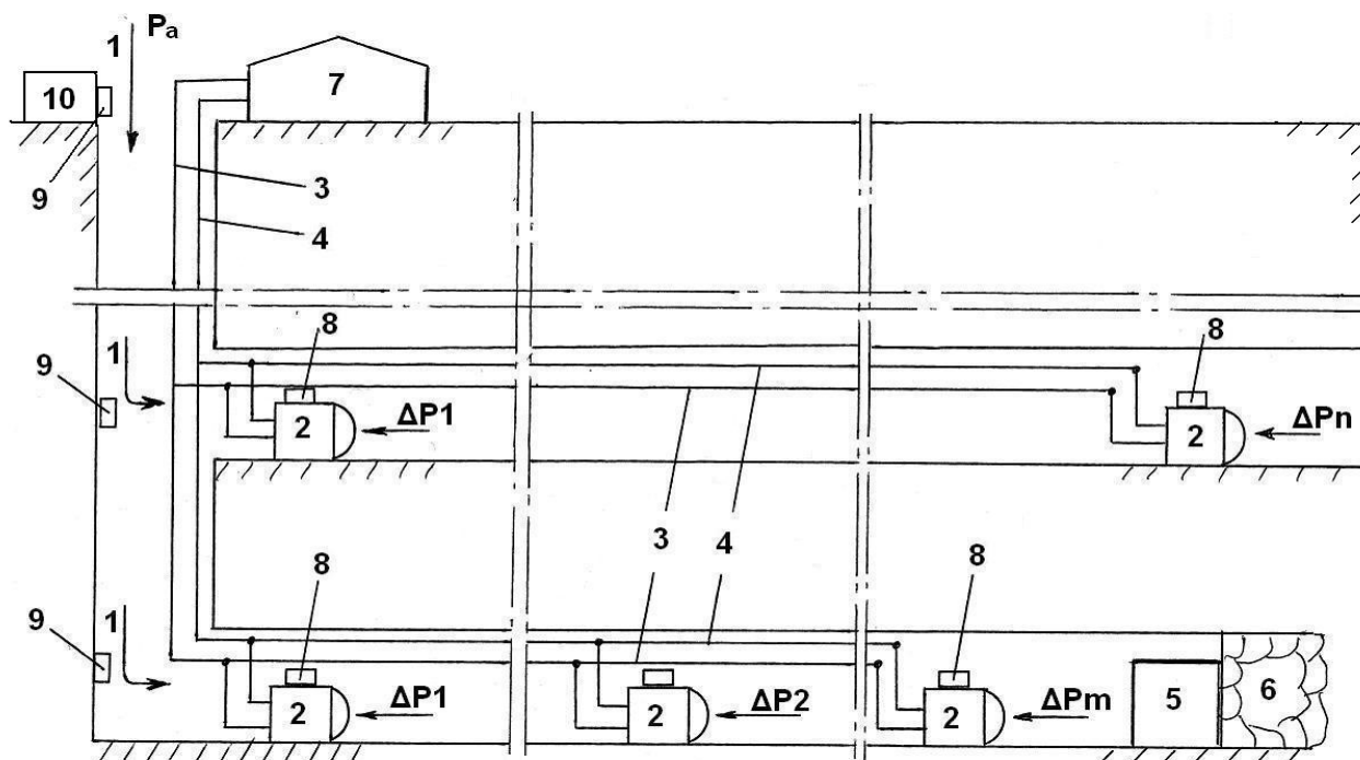
Рис.1- Блок-схема системы обеспечения безопасности угольных шахт
